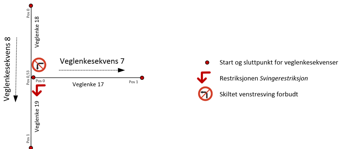
Figur 32 Eksempel på svingerestriksjon med retning
