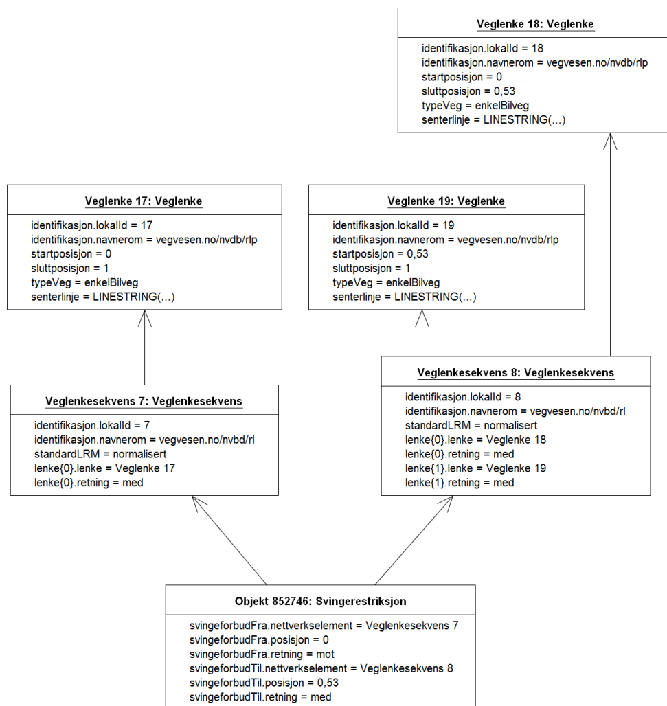
Figur 33 Eksempel på svingerestriksjon med retning
