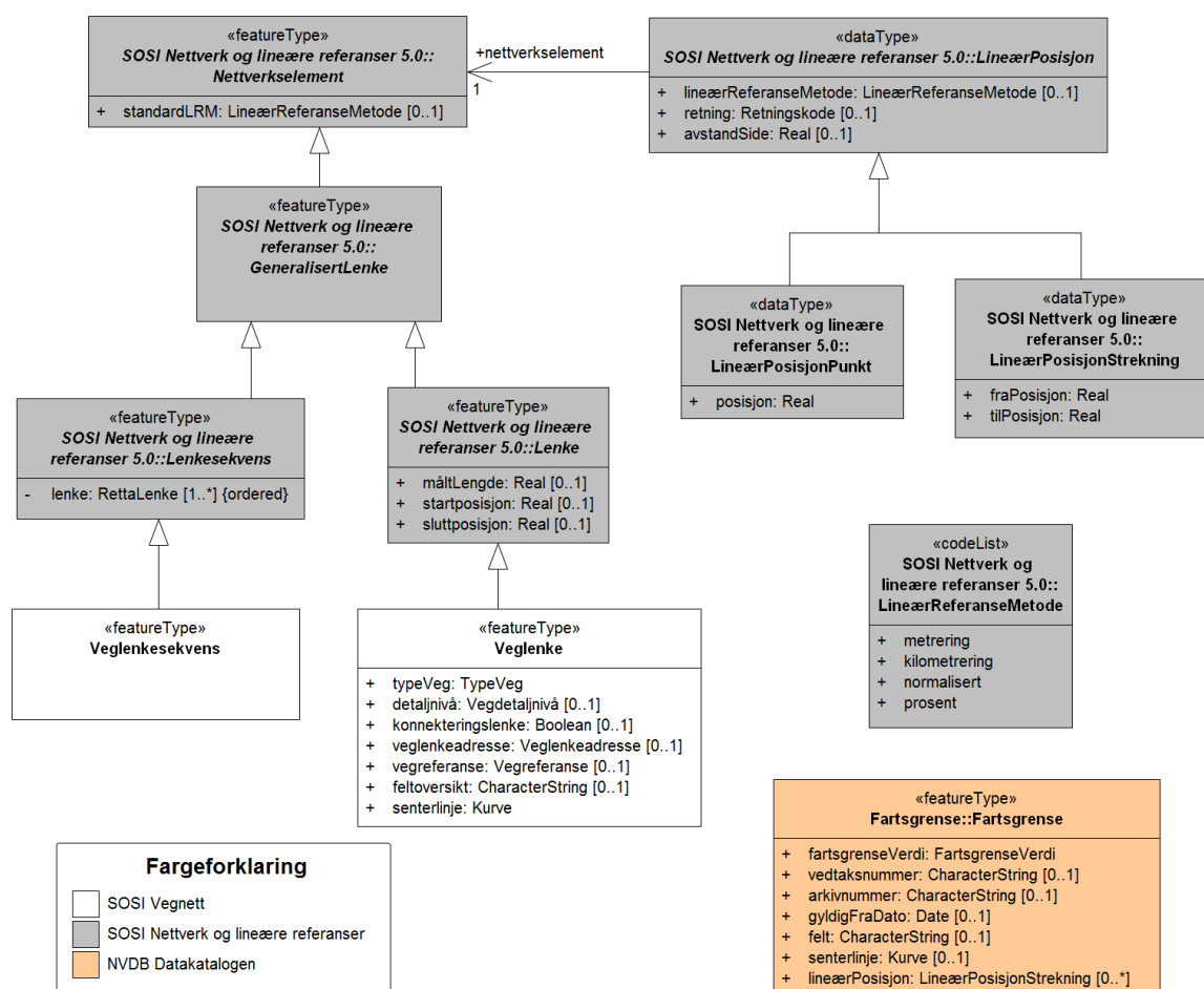
Figur 27 Stedfesting av objekter i vegnettet
