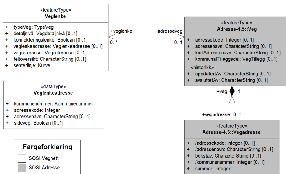
Figur 19 Veglenkeadresse og forholdet til offisielle adresser
