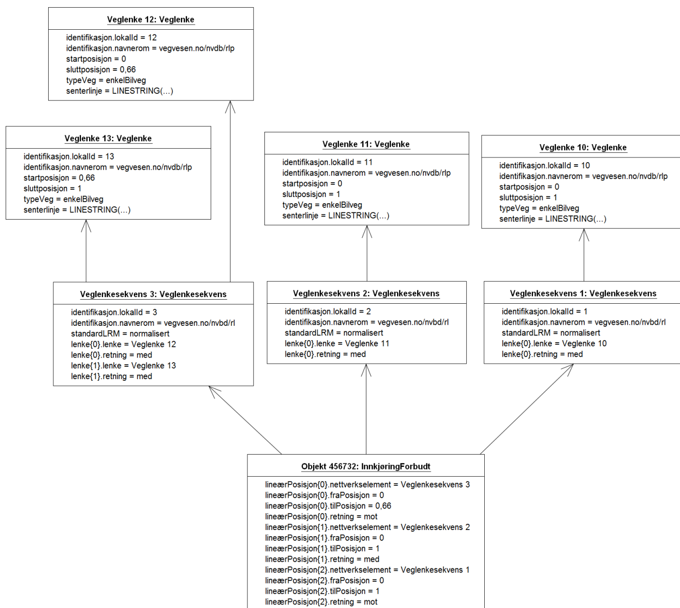
Figur 31 Eksempel på instans som er stedfestet med retning
