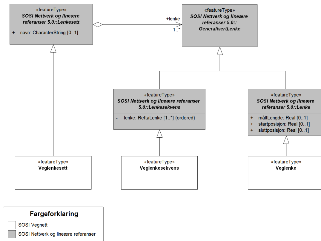
Figur 26 Veglenkesett
