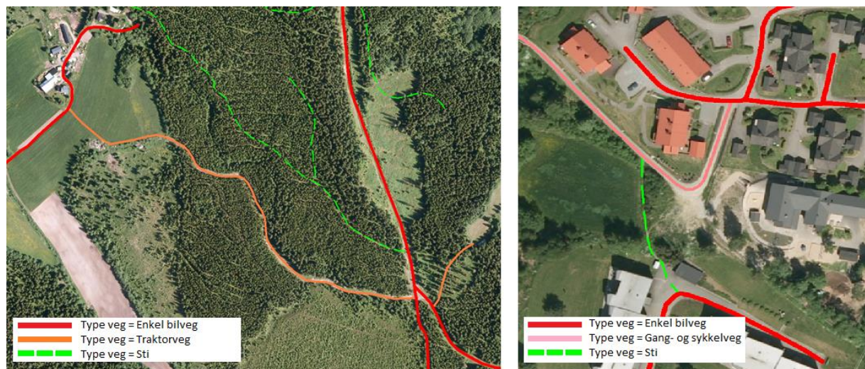
Figur 7 Vegtyper
