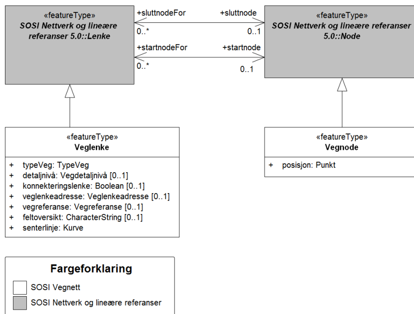
Figur 24 Vegnode
