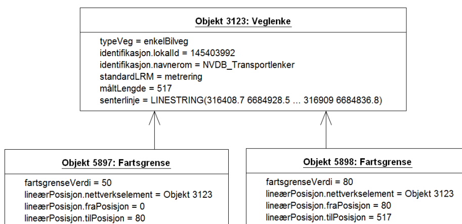
Figur 29 Eksempler på instanser av Veglenke og Fartsgrense med lineære referanser
