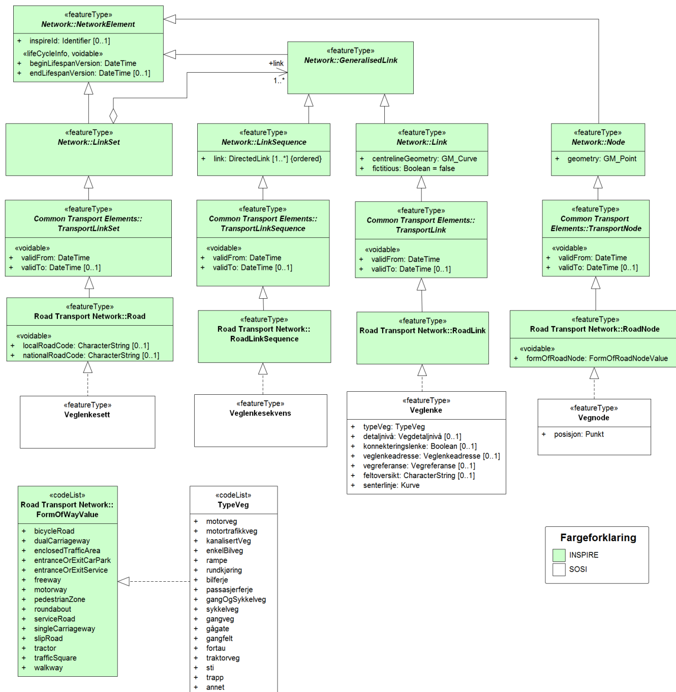
Figur 35 Realisering av INSPIRE Road Transport Networks
