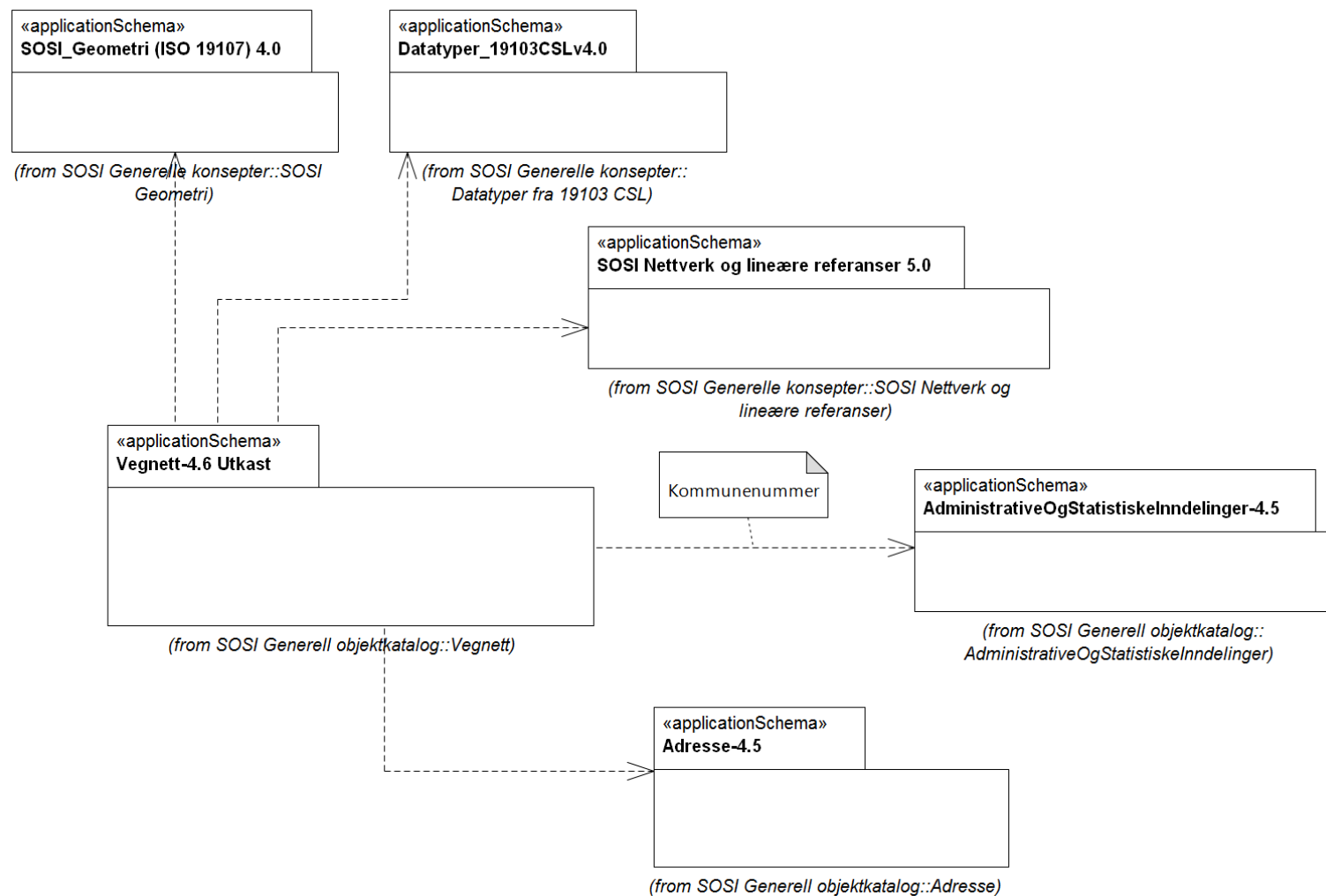
Figur 36 Pakkeavhengighet
