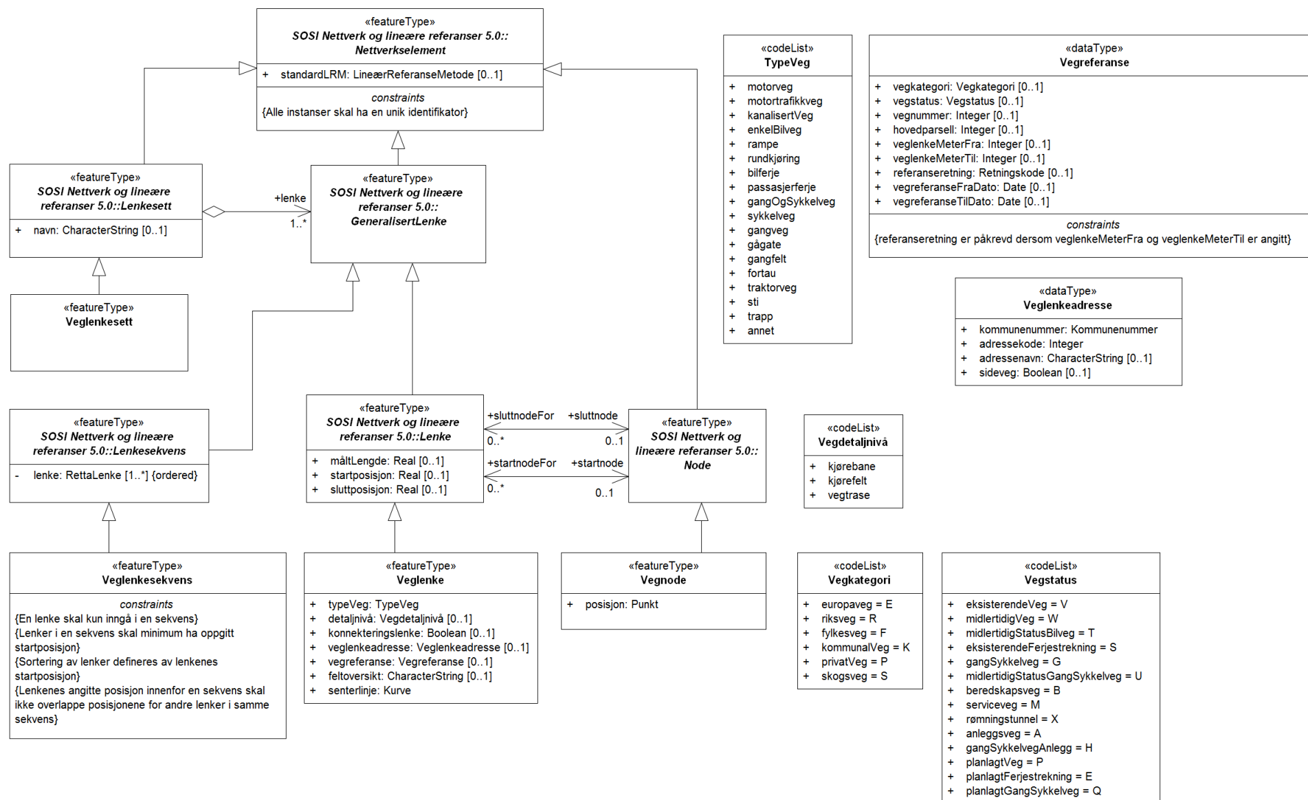
Figur 37 Hoveddiagram
