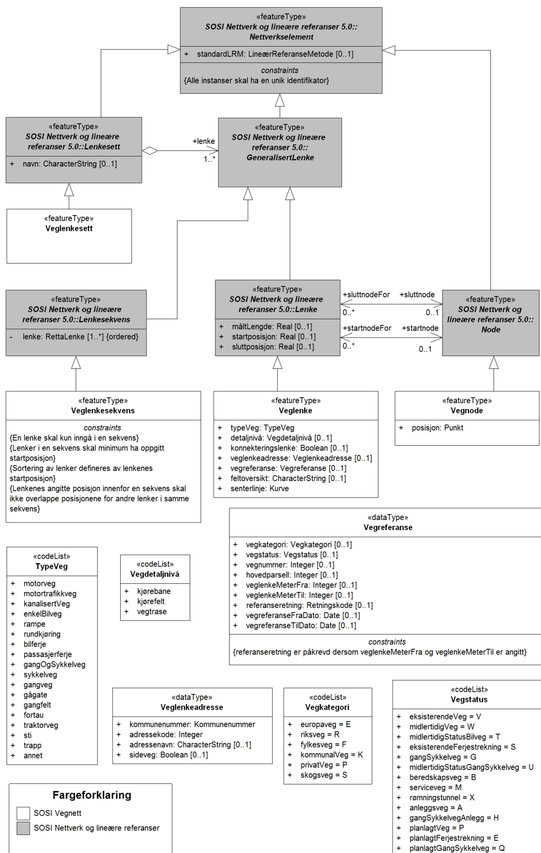
Figur 1 Fullstendig modell
