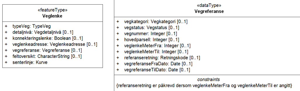
Figur 20 Vegreferanse
