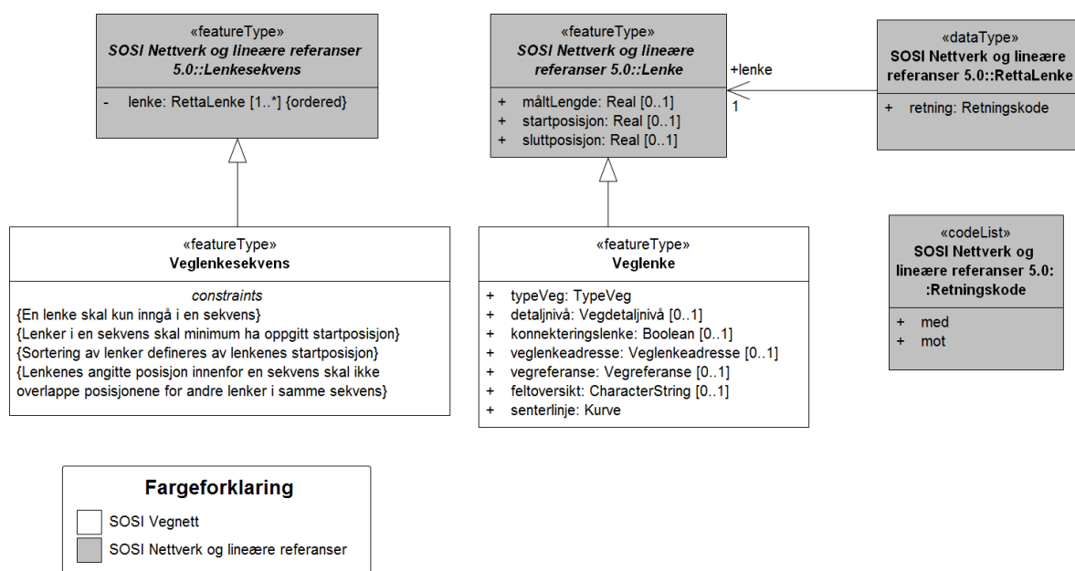
Figur 25 Veglenkesekvens
