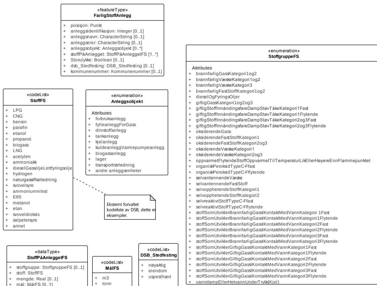
Figur 3 FarligStoffAnlegg
