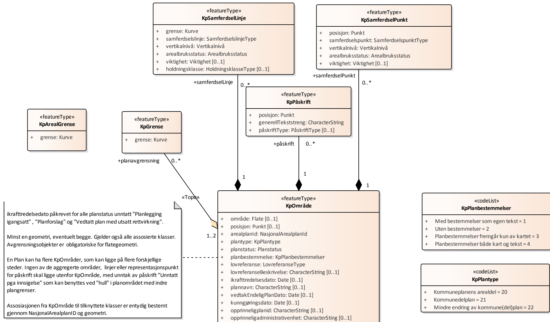
Figur 11: Modell felles for pbl. 1985 og pbl. 2008
