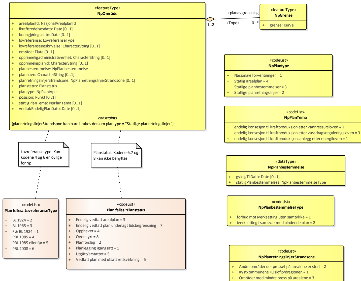
Figur 3 NasjonalePlanbestemmelser
