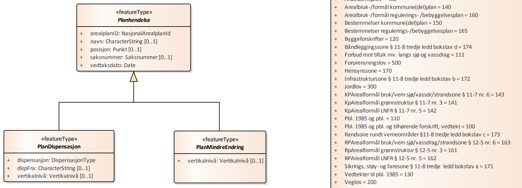
Figur 23 Planhendelser - hovedskjema
