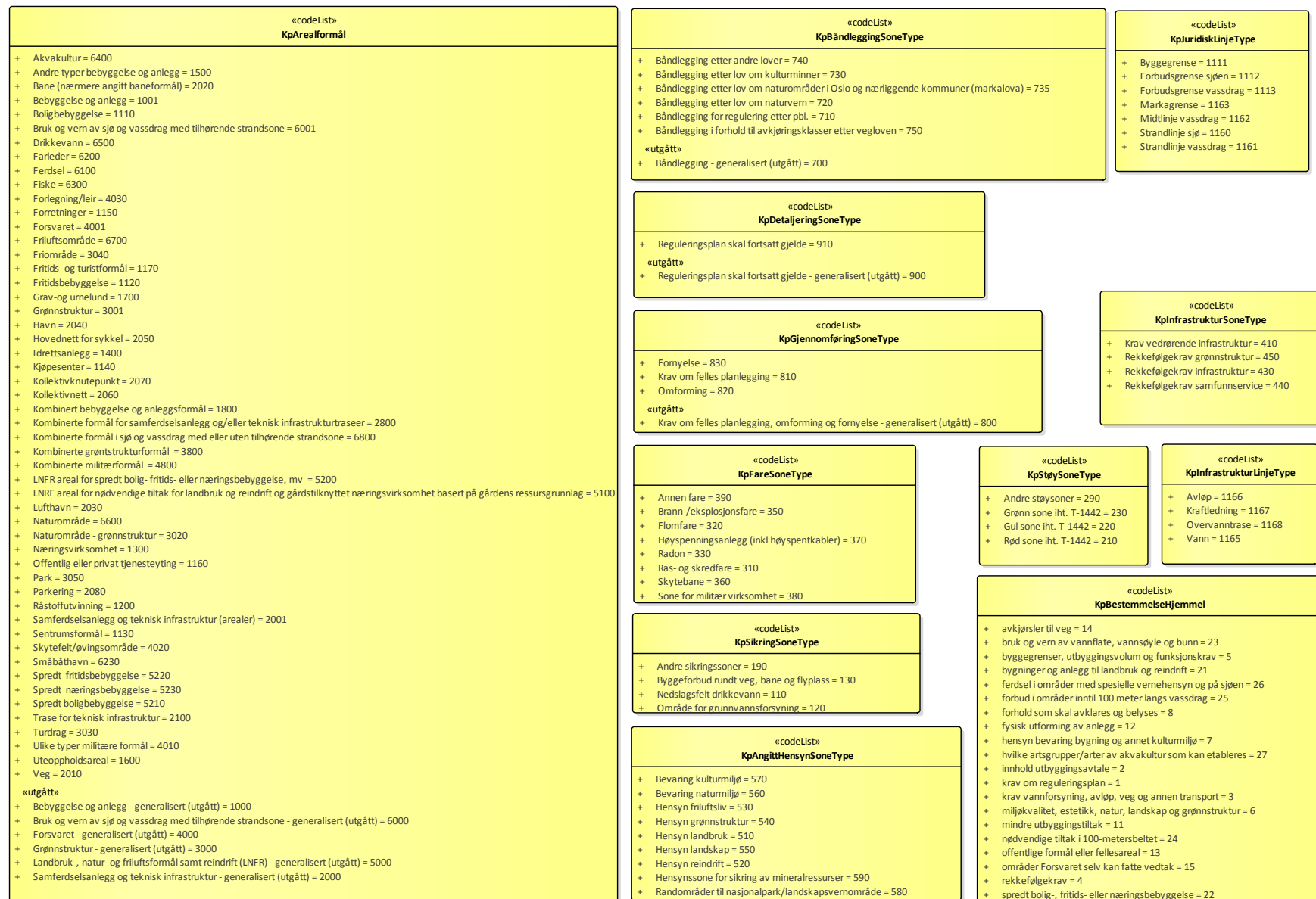
Figur 13 Kp 2008 Kodelister
