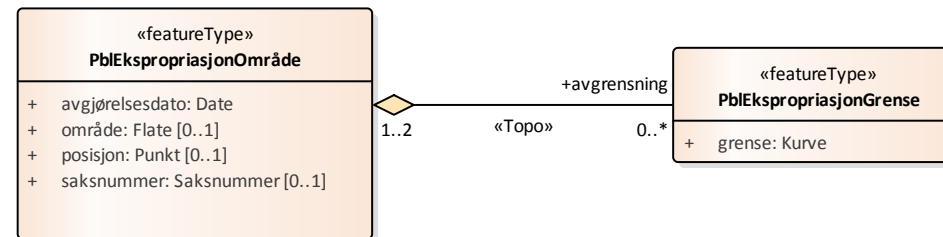
Figur 26 Hovedskjema Ekspropriasjon
