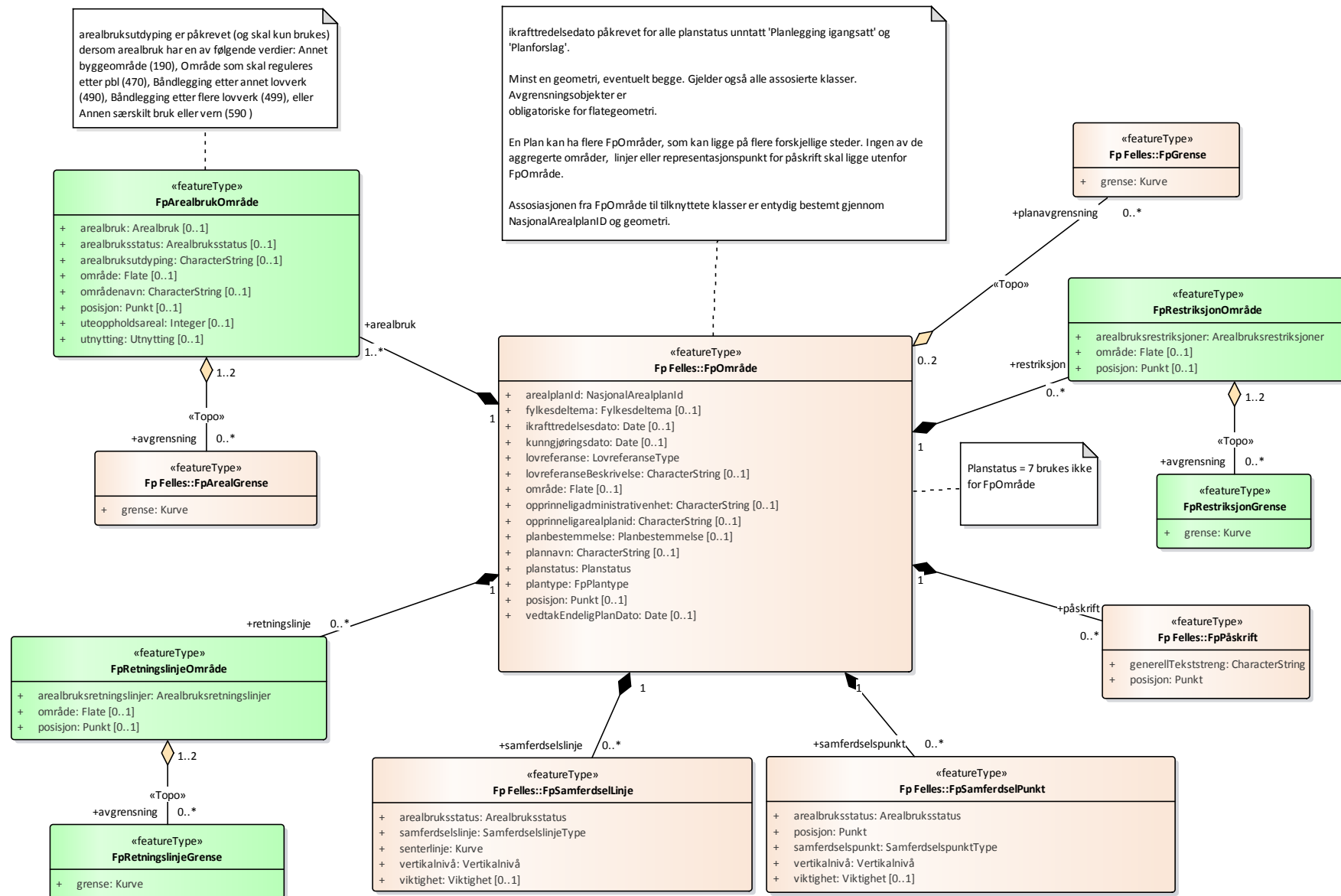
Figur 8 Fp 1985 Hovedskjema
