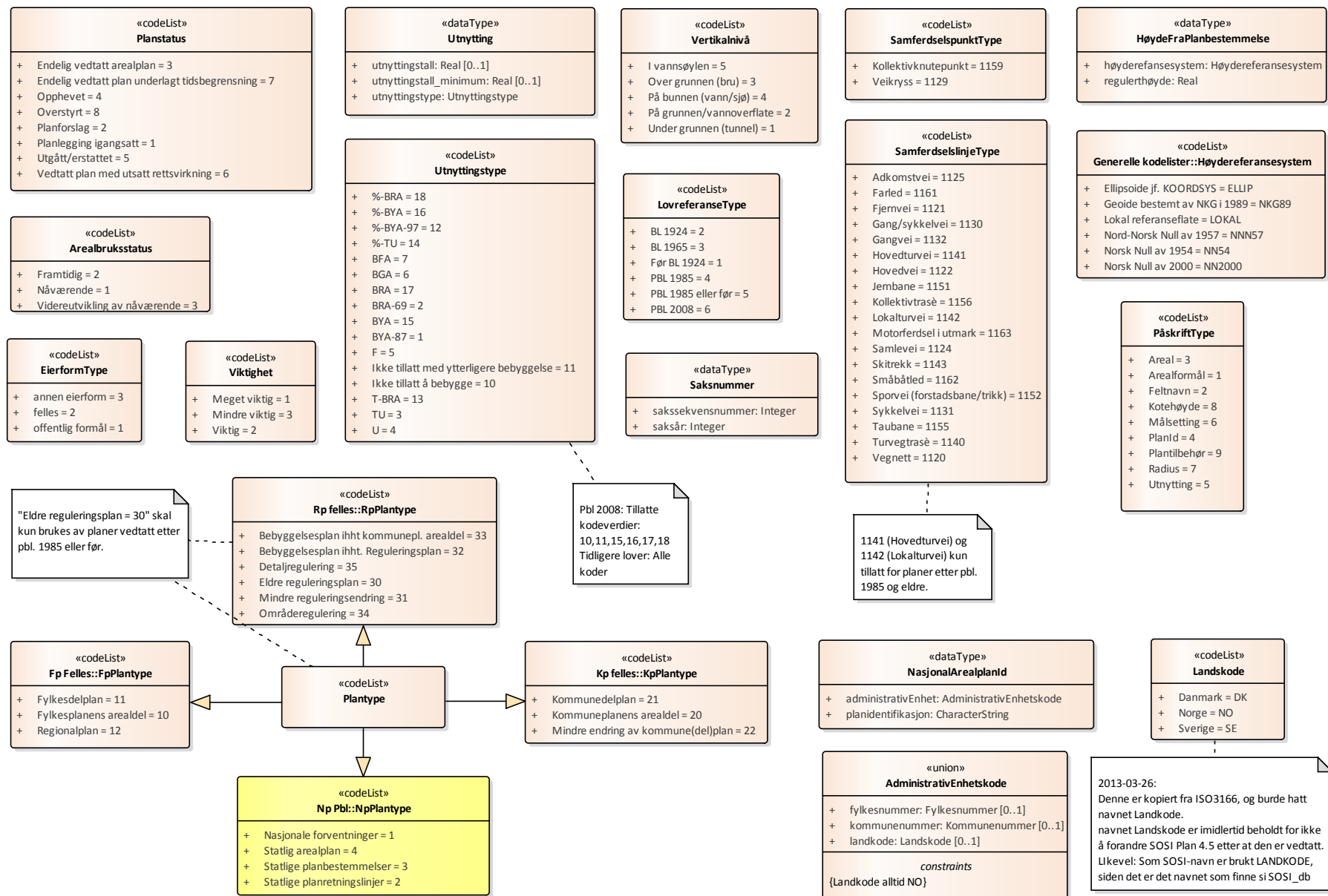
Figur 31 KodelisteGenerell
