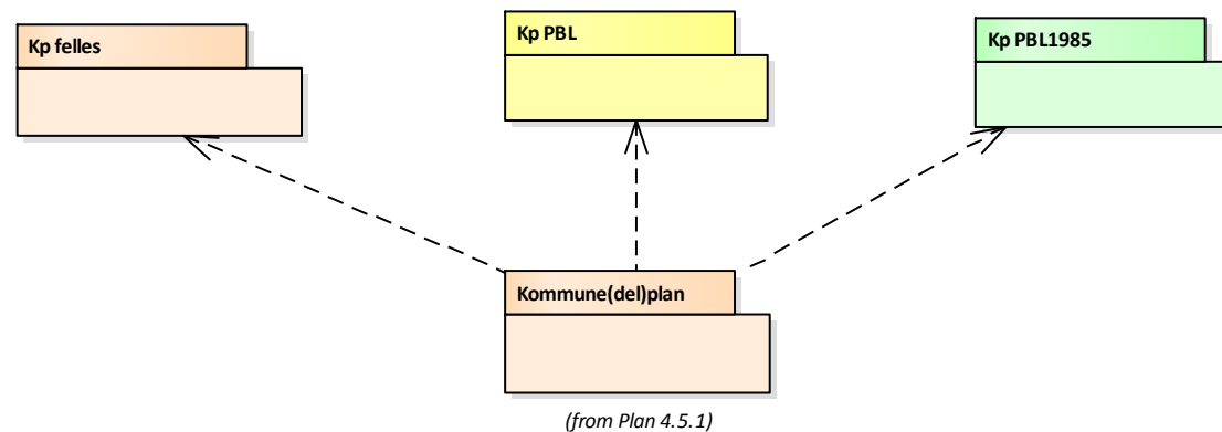
Figur 9 Kp pakkeoversikt
