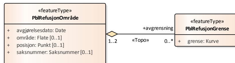
Figur 27 Hovedskjema Refusjon
