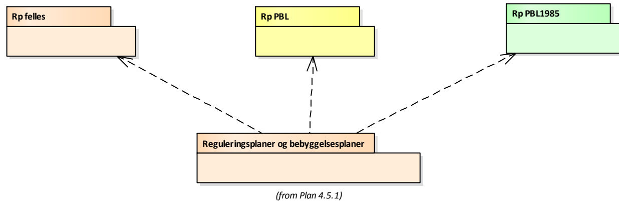
Figur 16 Rp pakkeoversikt
