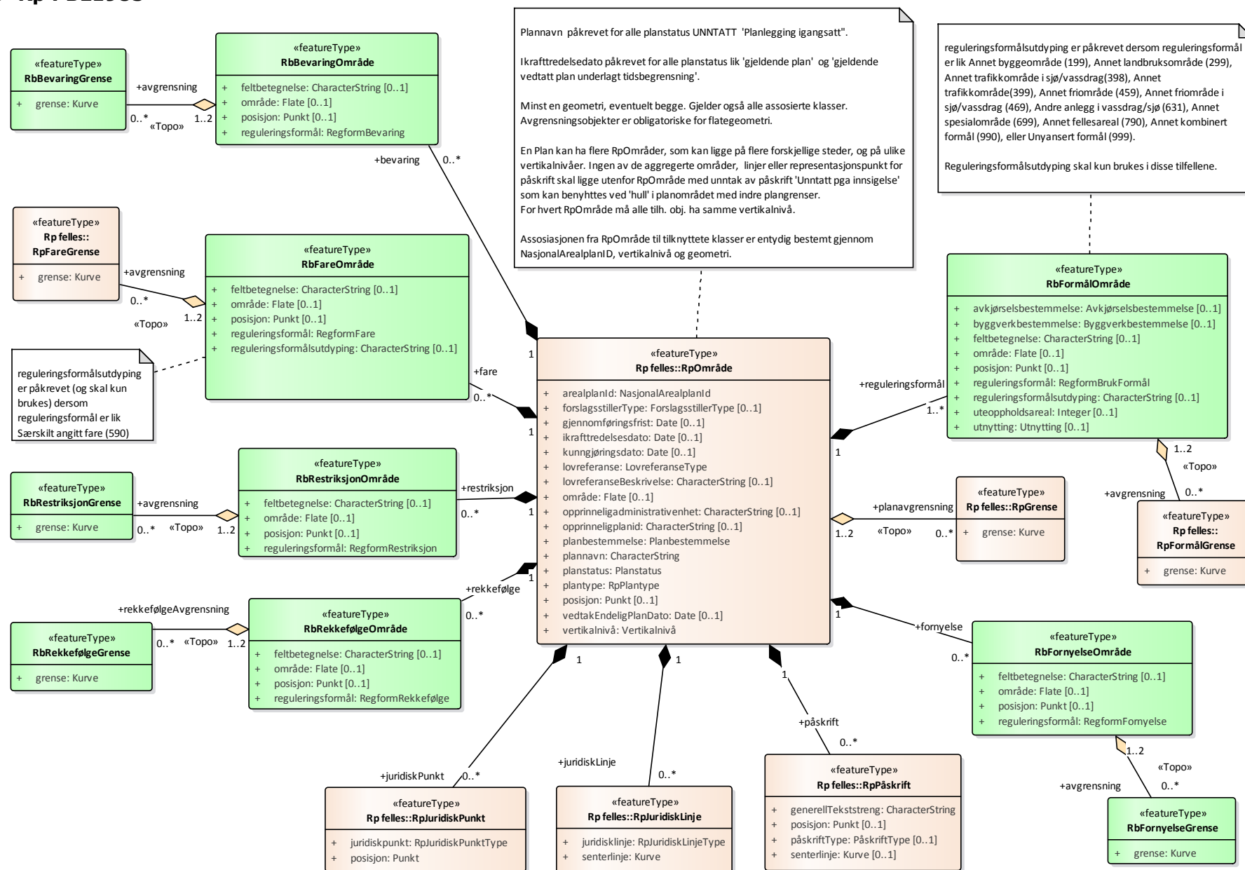
Figur 21 Rp 1985 hovedskjema
