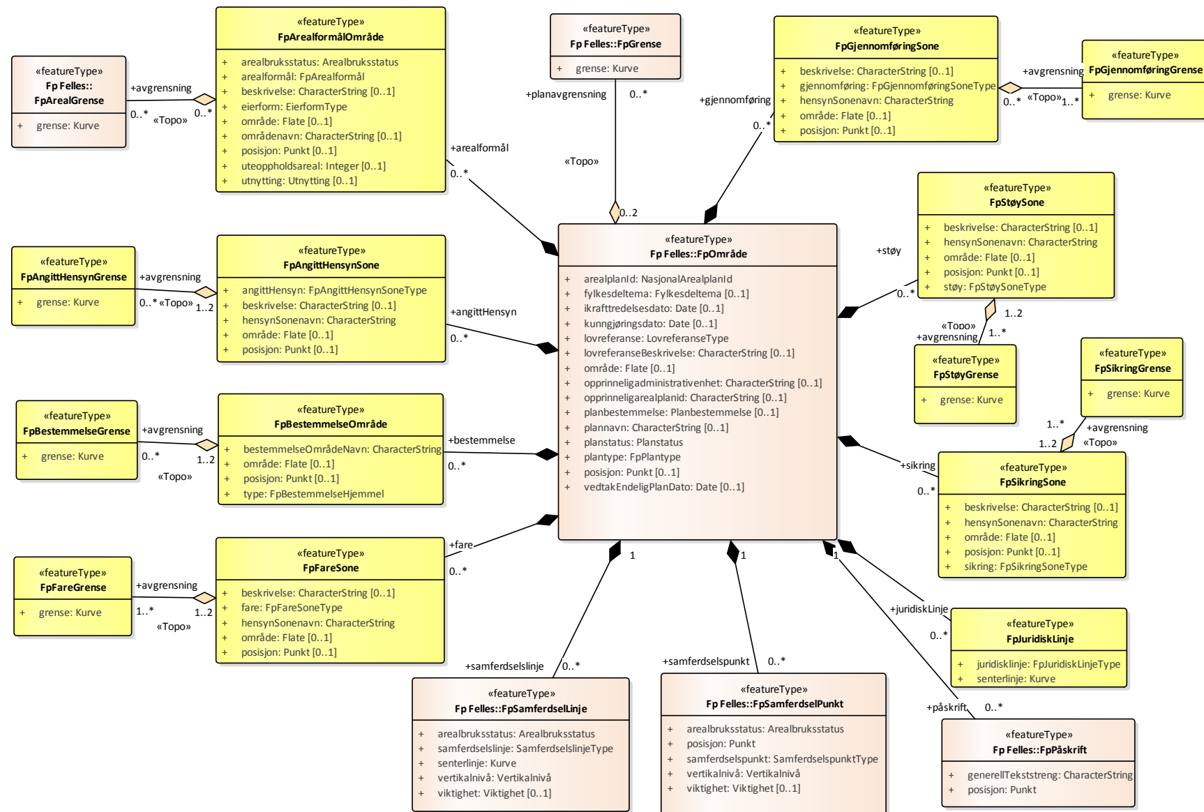
Figur 6 Fp Hovedskjema
