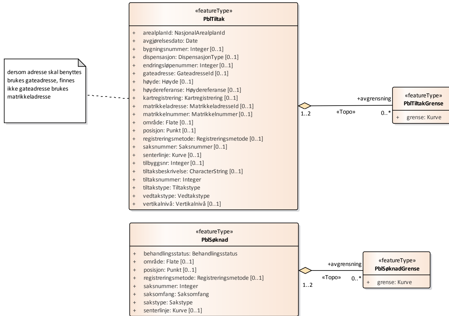
Figur 28 EnkeltSaker Hovedskjema
