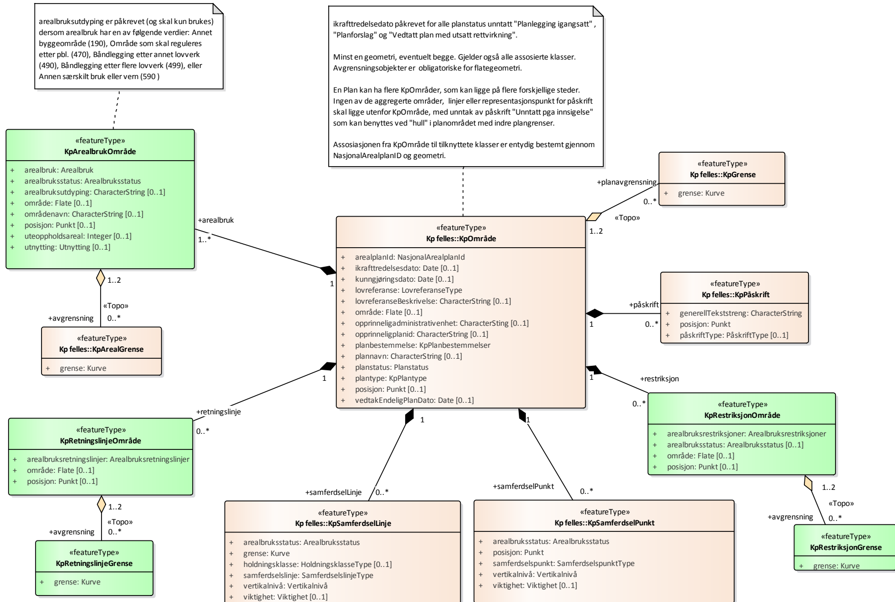
Figur 14 Kp 1985 Hovedskjema
