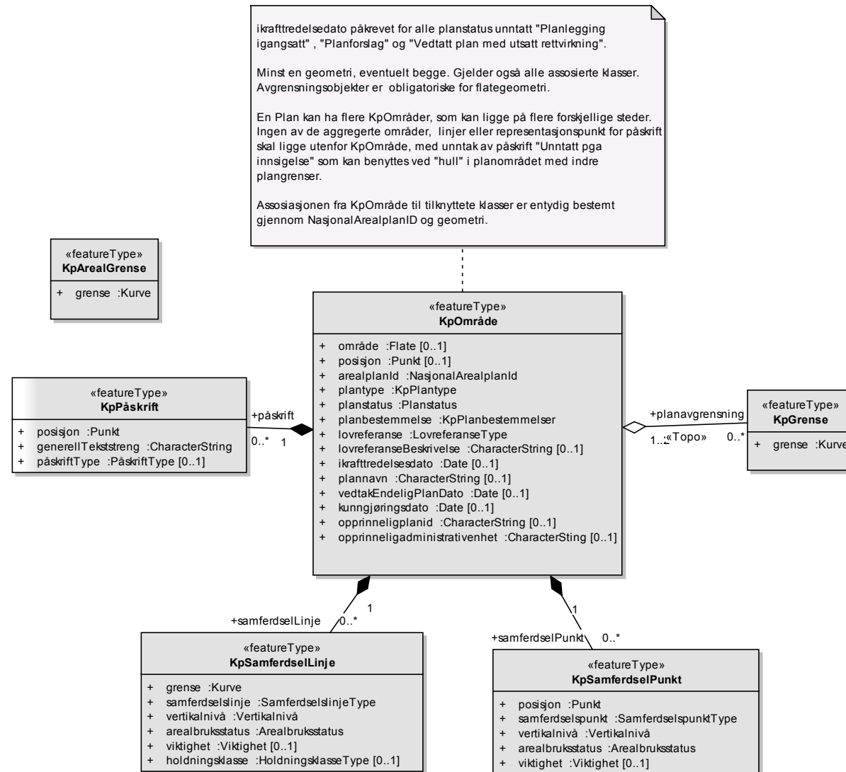
Figur 10 Modell felles for pbl. 1985 og pbl. 2008
