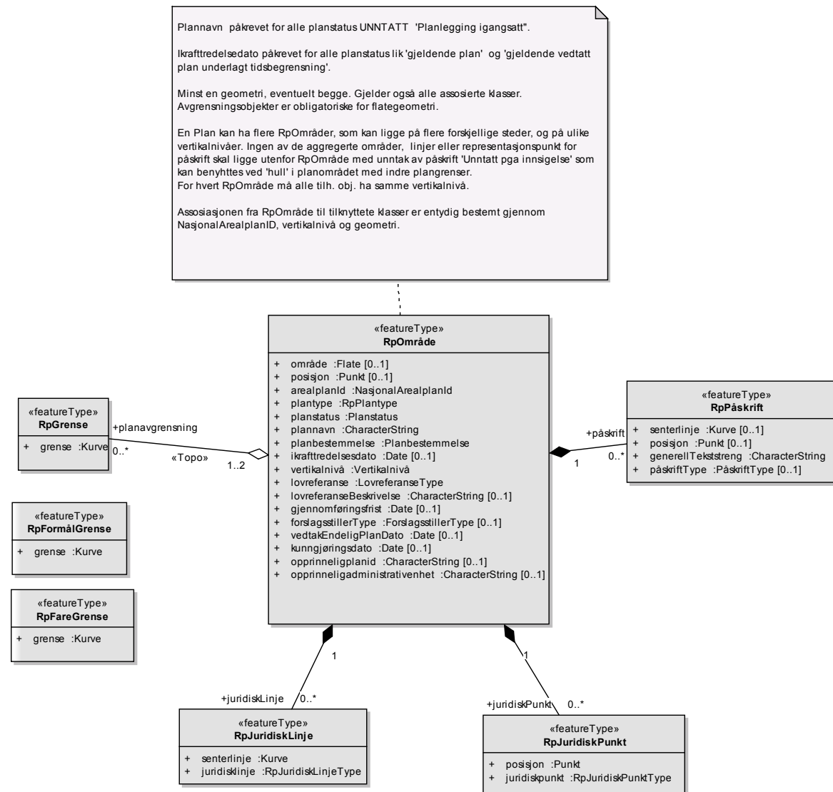
Figur 17 Rp Felles modell for pbl. 1985 og pbl. 2008
