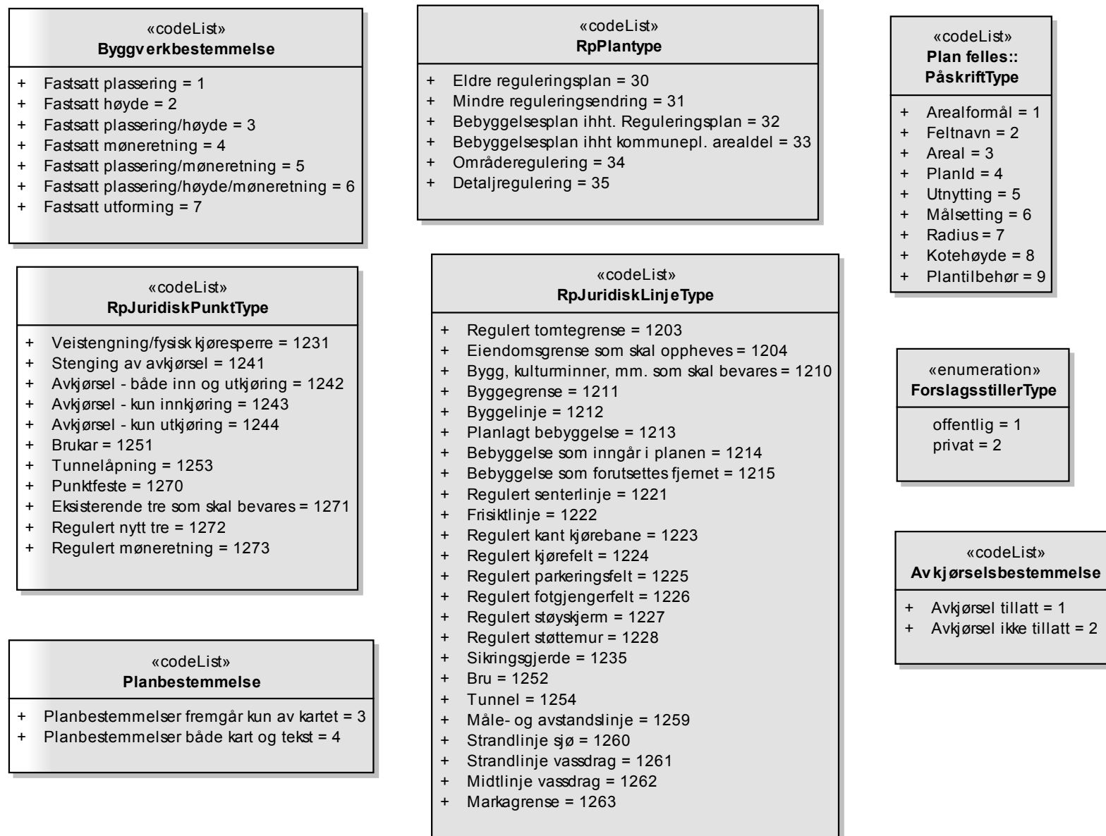
Figur 18 Rp Felles kodelister pbl. 1985 og pbl. 2008
