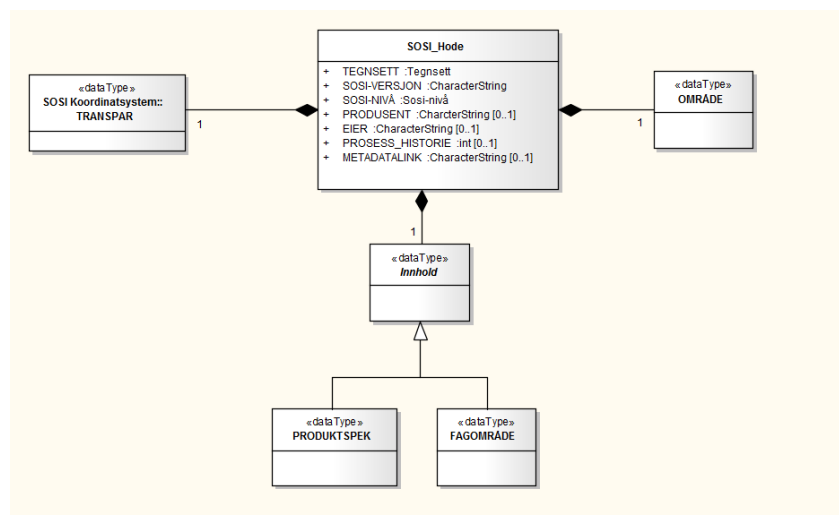
Figur 31 SOSI-hodet (forslag til illustrasjon av oppbygging)
