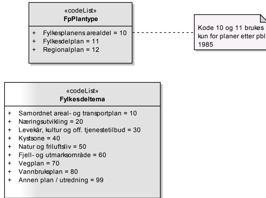
Figur 5 Fp Felles Kodelister
