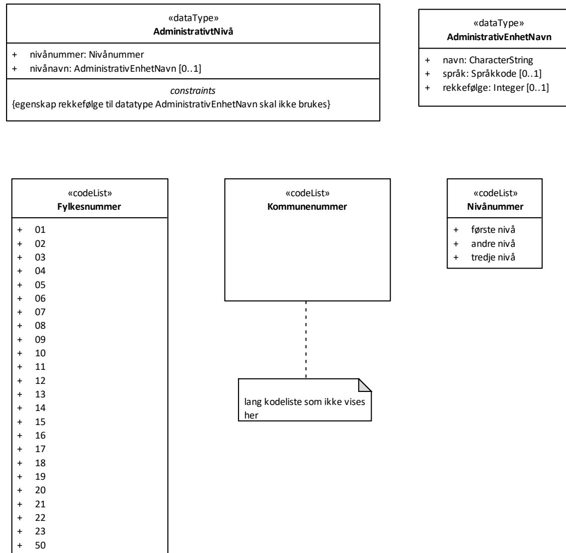
Figur 9 Datatyper og kodelister
