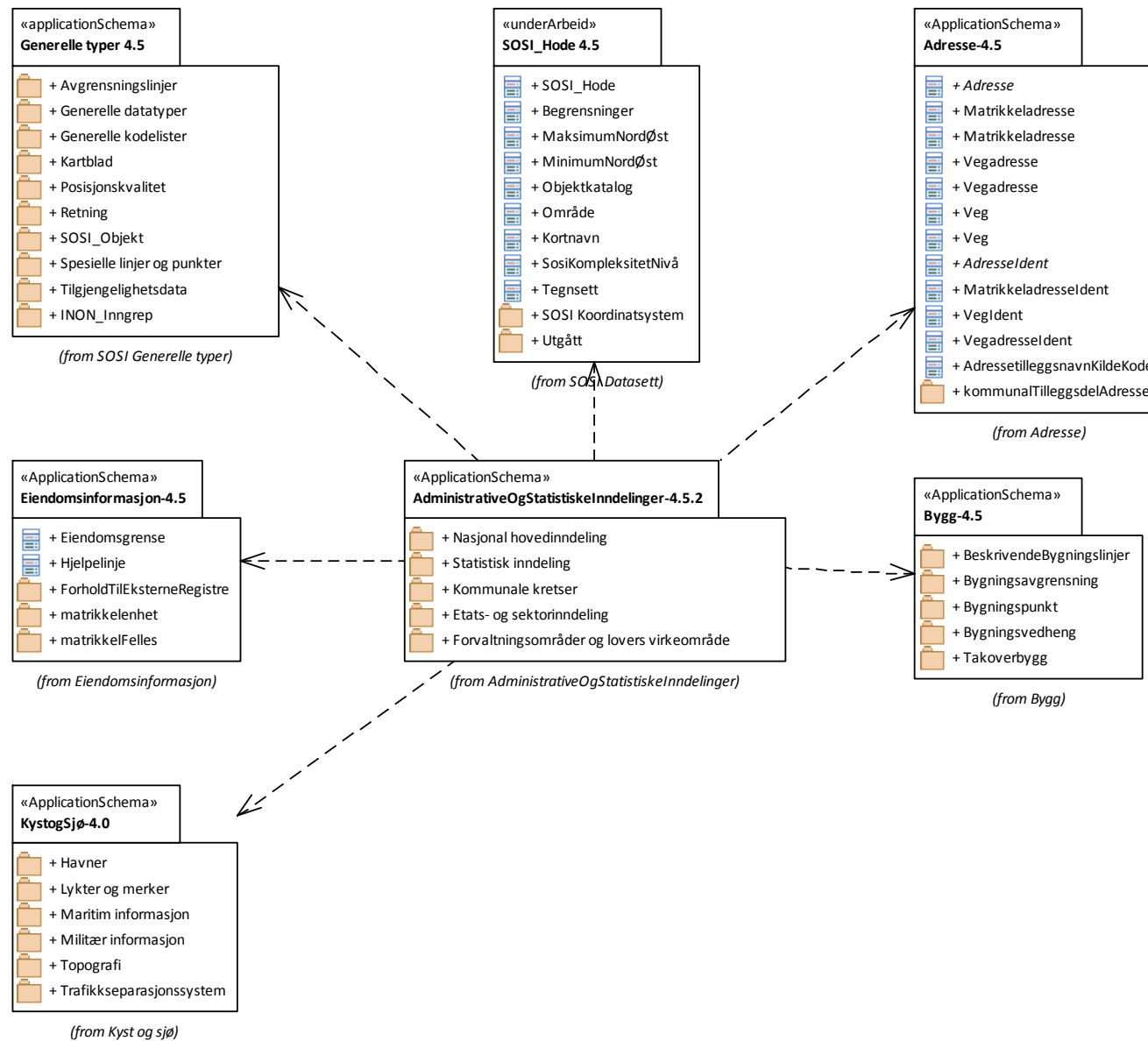
Figur 1 Pakkeavhengighet
