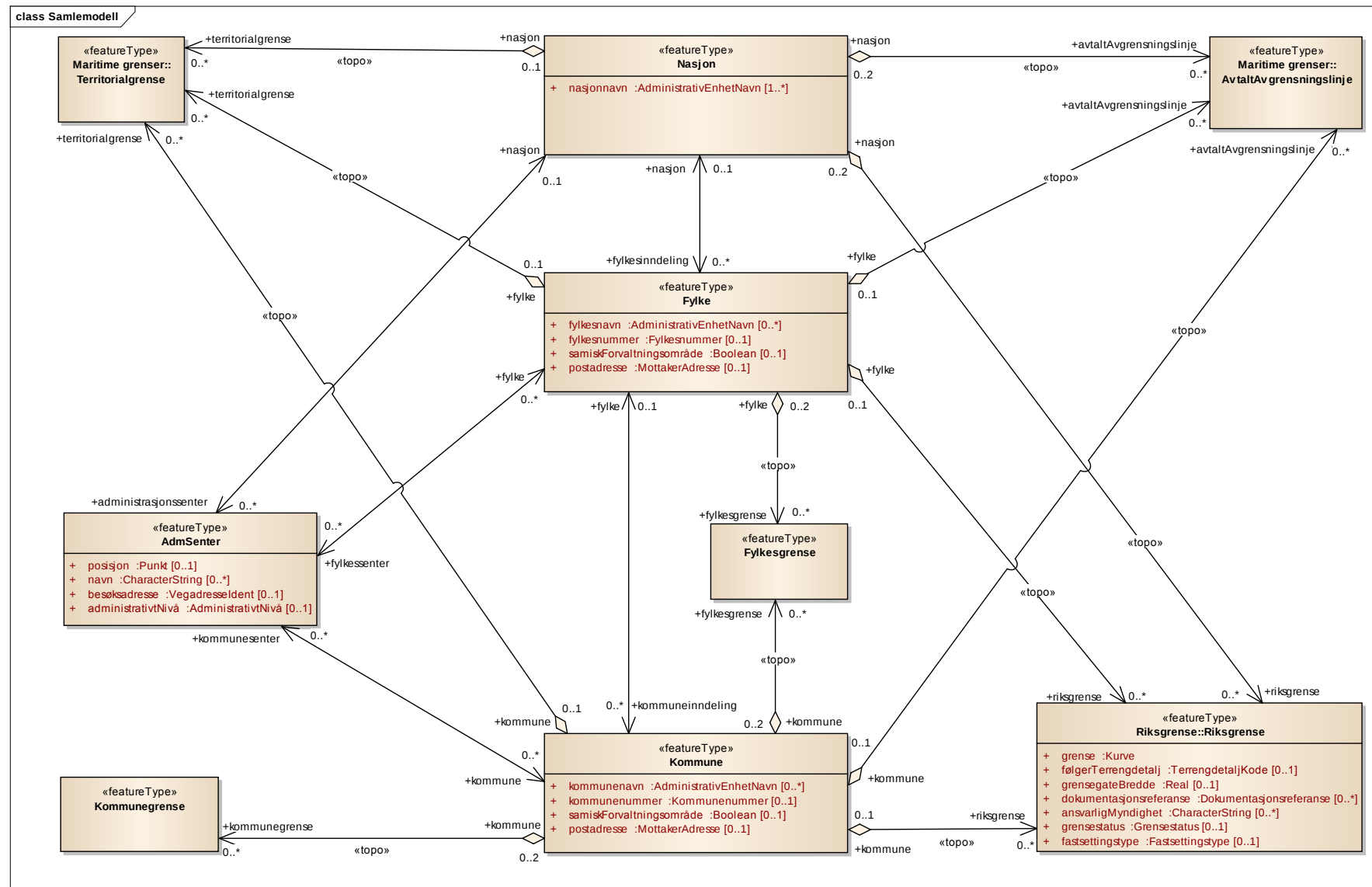
Figur 2 Samlemodell
