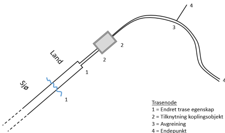
Figur 2: Trasenoder angir start- og sluttpunkt på en traseeksjon
