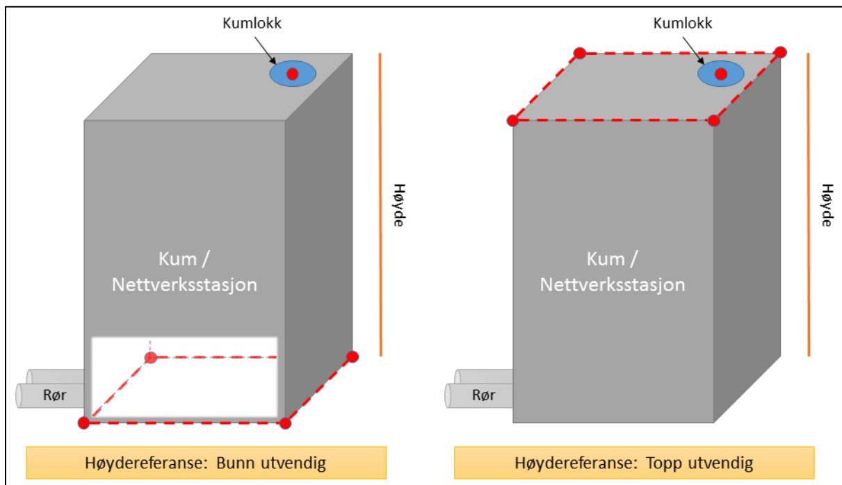
Figur 22: Alle ikke sirkulære koplingsobjekt skal registreres med hjørnekoordinater, primært bunn (alternativt topp), og høyde angivelse. Koplingsobjektets adkomst, her illustrert i form av kumlokk, skal stedfestes med senterpunkt for adkomsten.
