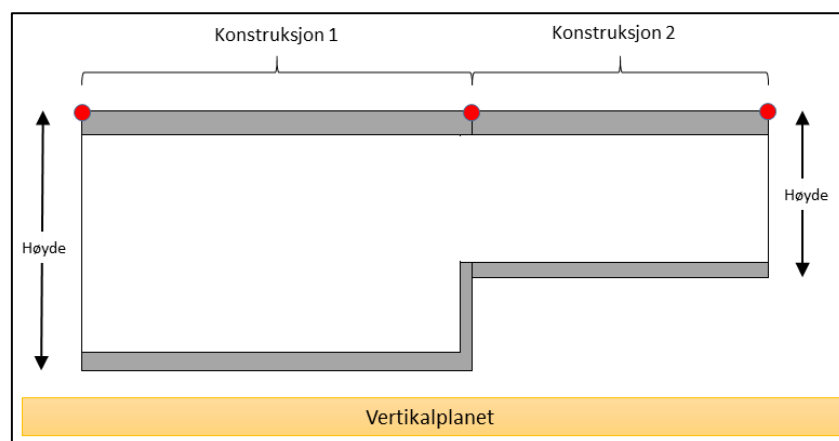
Figur 17: Nytt stedfestet punkt skal registreres når det skjer en endring av objektets bredde eller høyde. Konstruksjon 1 og 2 registreres som to objekter fordi endring i angitt høyde overskrider kravet til maksimalt tillatt avvik fra ytre avgrensing i vertikalt plan.
