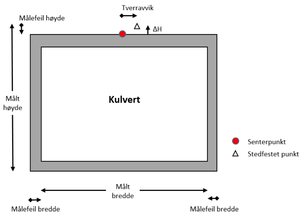
Figur 8: Figuren viser tverrsnitt av kulvert påført eksempler på feil for de feiltyper som angår stedfesting av tverrsnittet.
