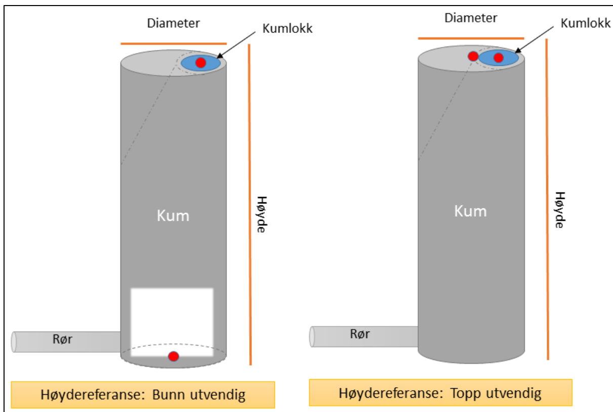
Figur 21: Alle sirkulære koplingsobjekt skal registreres med senterpunkt samt diameter og høyde. Z-verdi skal registreres på bunn utvendig kum, - dersom ikke registrering av topp utvendig kum er avtalt. Koplingsobjektets adkomst, her illustrert i form av kumlokk, skal stedfestes med senterpunkt for adkomsten.
