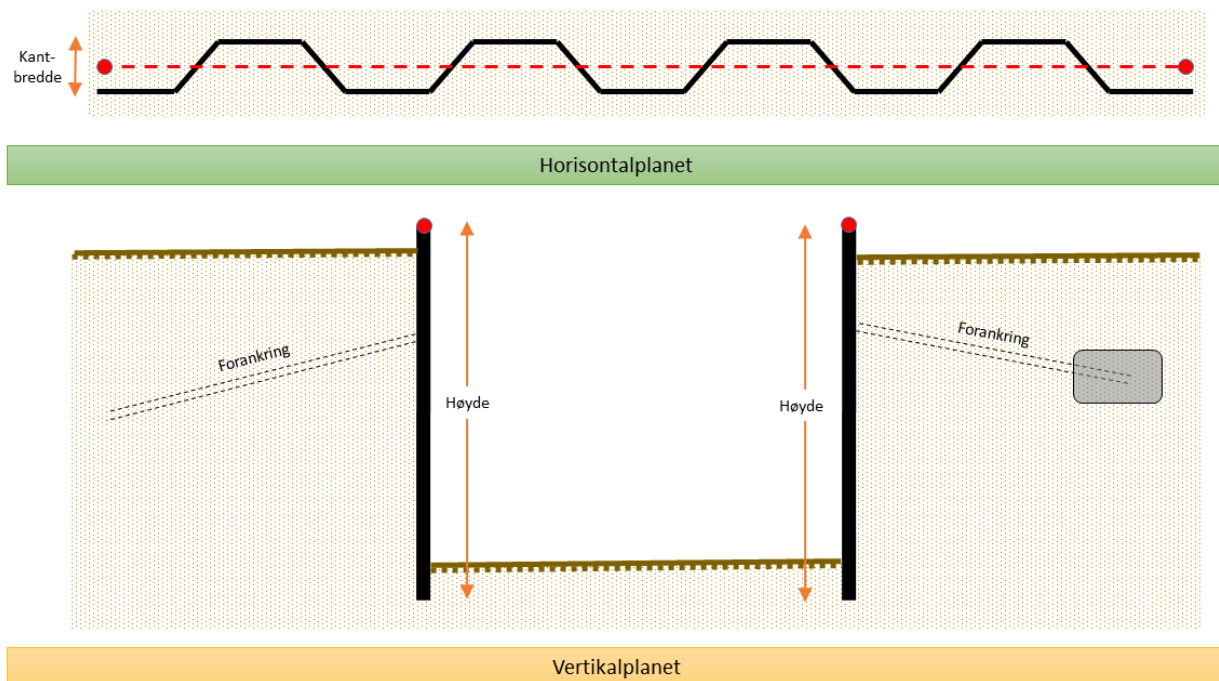
Figur 27: Eksempel på stedfesting av vertikal spuntvegg i horisontal- og vertikalplanet. Figuren viser eksempel på to varianter av forankringsstag.
