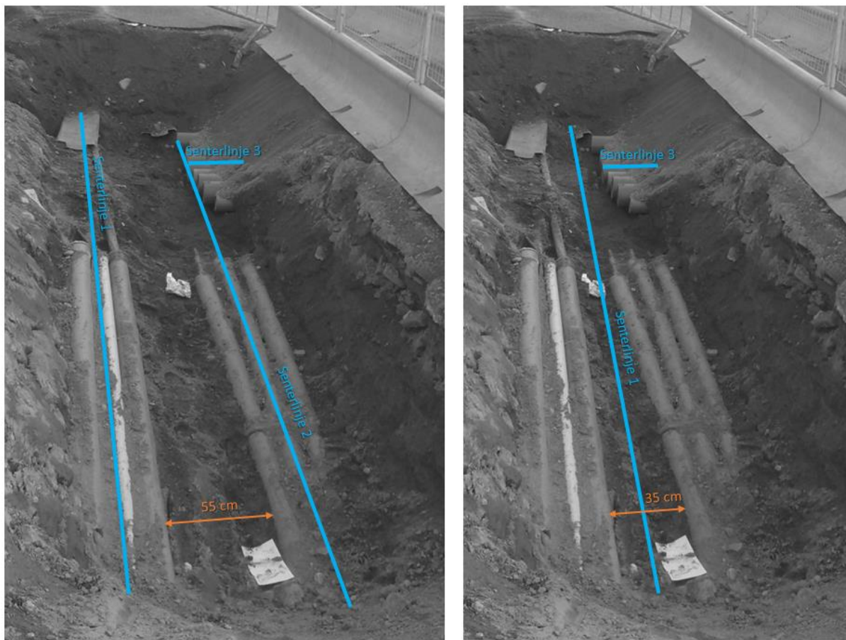
Figur 9: Dersom avstanden mellom to ledningsgrupper i grunnen er større enn 40 centimeter i grunnriss og/eller høyde, innenfor områdetype 1, skal hver av ledningsgruppene registreres med en senterlinje (ledningstrase). Dersom avstanden er under 40 centimeter er det opp til ledningseier å avgjøre om man ønsker å registrere en eller flere senterlinjer (ledningstraseer).
