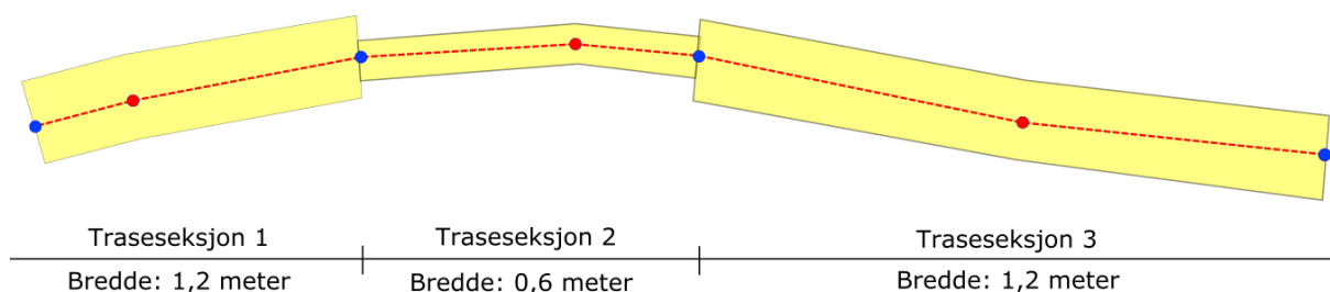
Figur 10: Dersom bredden i en ledningstrase endres får vi en ny traseseksjon. Start- og slutt punktet i hver av traseseksjonene er en trasenode (blå punkt). Røde og blå punkt markerer stedfestede punkt på senterlinjen.
