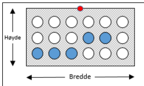
Figur 6: En ledningstrases ytre avgrensning kan stedfestes ved hjelp av senterlinje, høyde og bredde.
