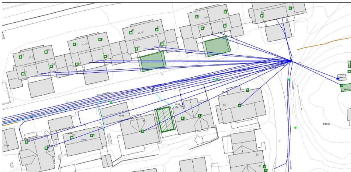
Figur 26: Eksempel på «Ledningskart» med rette linjer mellom koplingsobjekt og terminering hos abonnent. Her må det påvises hvor kablene går dersom det skal graves mellom husrekke.
