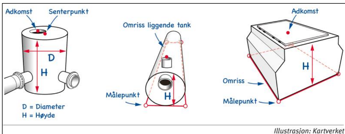
Figur 20: Eksempler på koplingsobjekt. Fra venstre: sirkulære i grunnriss, sirkulære i vertikalplanet, ikke sirkulære i grunnriss. Illustrasjon: Kartverket
