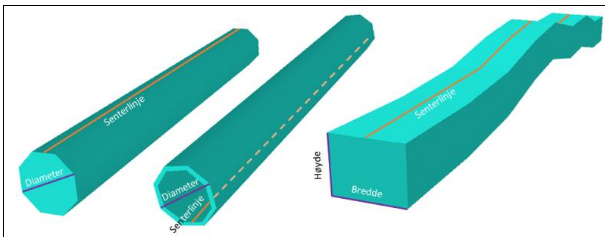
Figur 12: Alle ledningstraseer (enkeltledninger eller flere ledninger i samme trase) skal som minimum registreres med en senterlinje og ytre bredde og høyde eller diameter. I tillegg må høydereferanse angis.
