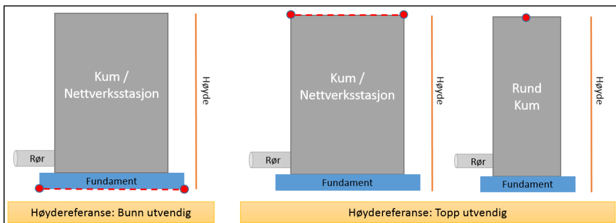
Figur 24: Stedfesting av koplingsobjekt med fundament
