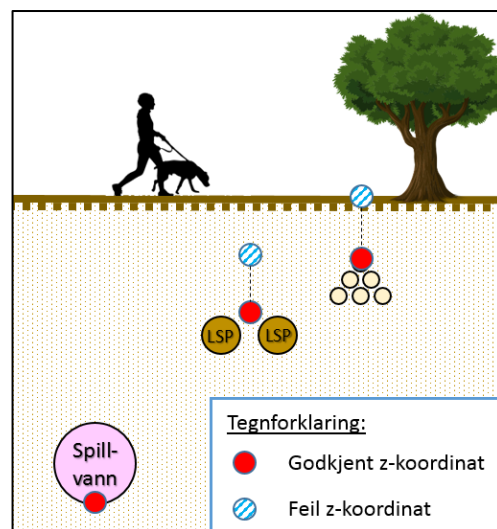
Figur 11: Registrert z-koordinat skal registreres på topp ledningstrase, mens bunn kan benyttes etter nærmere avtale.
