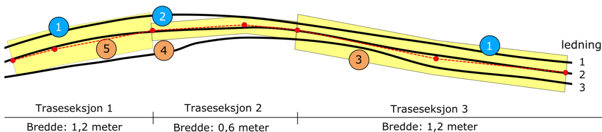
Figur 15: Eksempel med tre ledninger (1, 2 og 3) i en trase, og når stedfestet ledningstrase er innenfor eller utenfor tillatt maksimalt avvik.
