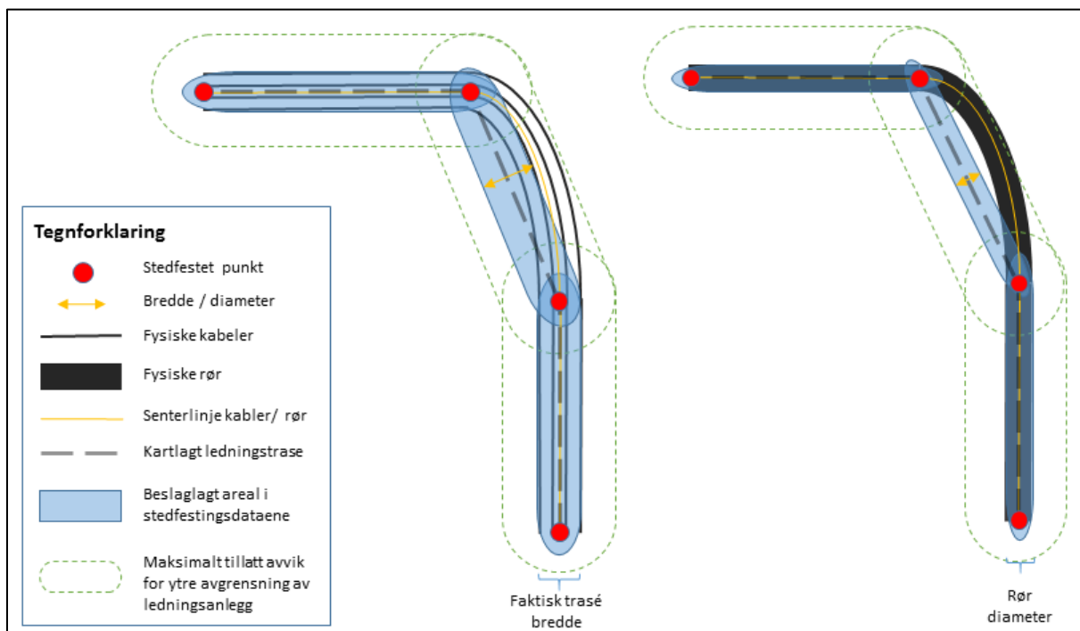
Figur 18: Eksempel som viser forholdet mellom beliggenhet til fysiske ledninger, stedfestet ledningstrase med bredde og maksimalt tillatt avvik i horisontalplanet. Merk at registrert beslaglagt areal kan være betydelig større enn det som objektet beslaglegger i virkeligheten
