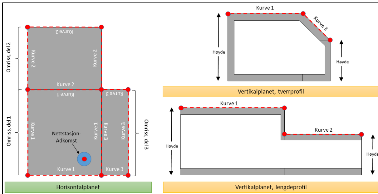
Figur 23: Stedfesting av nettverksstasjon med «irregulær geometri» kan stedfestes med flere delgeometrier
