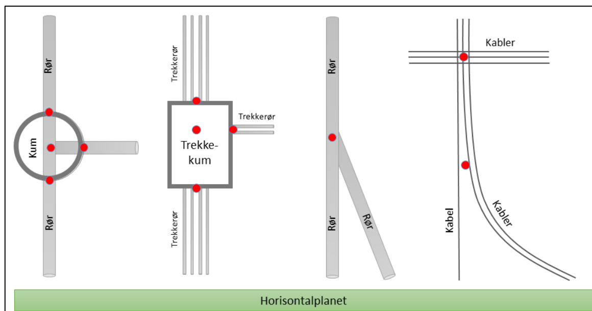
Figur 16: Målepunkt (rødt punkt) for ledninger som møtes eller går inn i et koplingsobjekt
