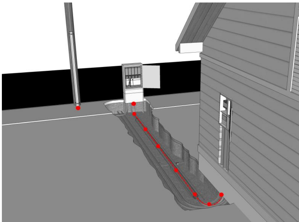
Figur 25: Rød punkt viser hvor langt registrering av ledninger i bakken går. Kilde: REN AS
